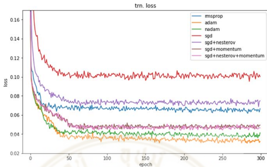
ภาพ 3.9 แสดงผลเปรียบเทียบการทำงานของ Optimizer ตัวต่างๆ
