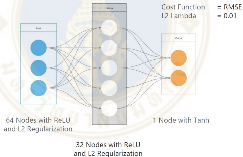
ภาพ 5.3 แสดงโครงสร้างของโครงข่ายประสาทเทียมที่ใช้ในการคาดการณ์ผลตอบแทนรายเดือนของตราสารทุนแต่ละตัว
