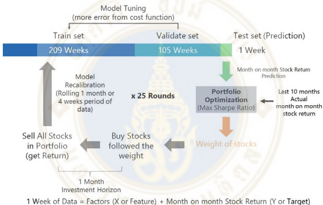
ภาพ 5.1 แสดงการขยับช่วงข้อมูลในแต่ละรอบการปรับแบบจำลองในการคาดการณ์ผลตอบแทนของตราสารทุนแต่ละตัว
