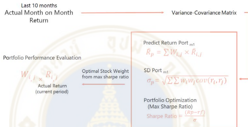
ภาพ 3.11 แสดงขั้นตอนการทำงานของวิธีการปรับพอร์ตโฟลิโอในการลงทุนโดยใช้ Mean-Variance Portfolio Optimization และเลือกน้ำหนักการลงทุนบนจุด Maximum Sharpe Ratio
