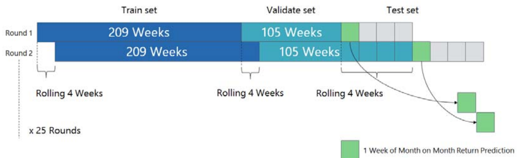
ภาพ 5.1 แสดงการขยับช่วงข้อมูลในแต่ละรอบการปรับแบบจำลองในการคาดการณ์ผลตอบแทนของตราสารทุนแต่ละตัว
