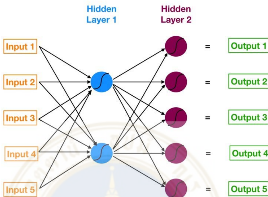
ภาพ 3.2 โครงสร้างแบบง่ายของการทำงานของโครงข่ายประสาทเทียม
